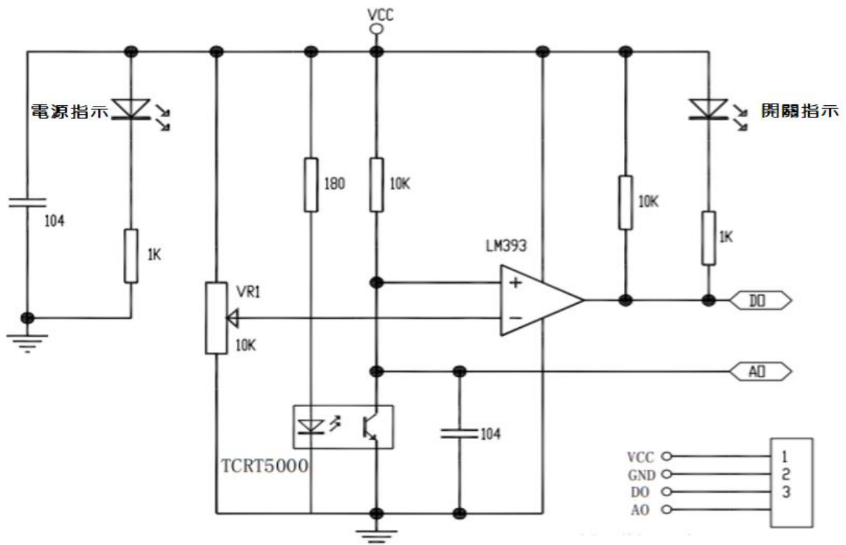
圖三：TCRT 5000 感測模組電路參考圖
